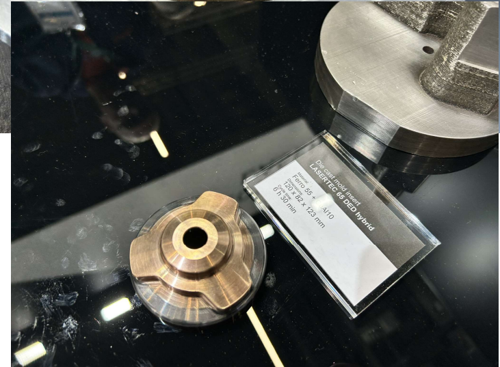
DMG Mori, DED Hybrid (CuAl10 + 316L / Ferro 55 + CuAl10)
